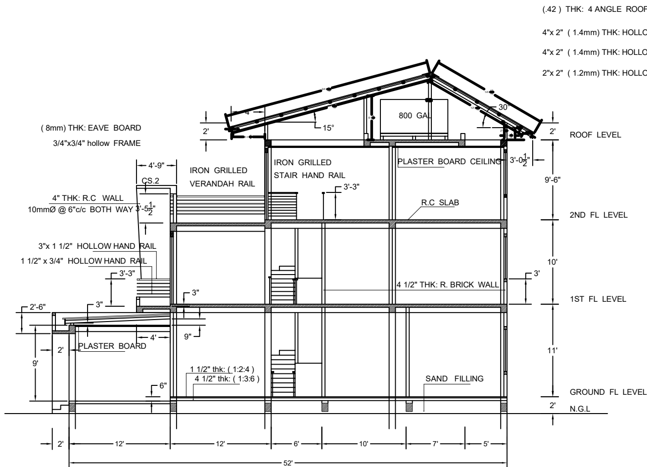
LONGITUDINAL SECTION
